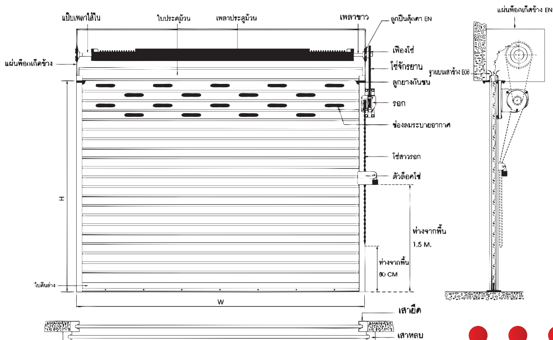
ตัวอย่างการติดตั้งประตูเหล็กม้วนระบบรอกโซ่ Rolling Shutter Installation of Chain Operation
