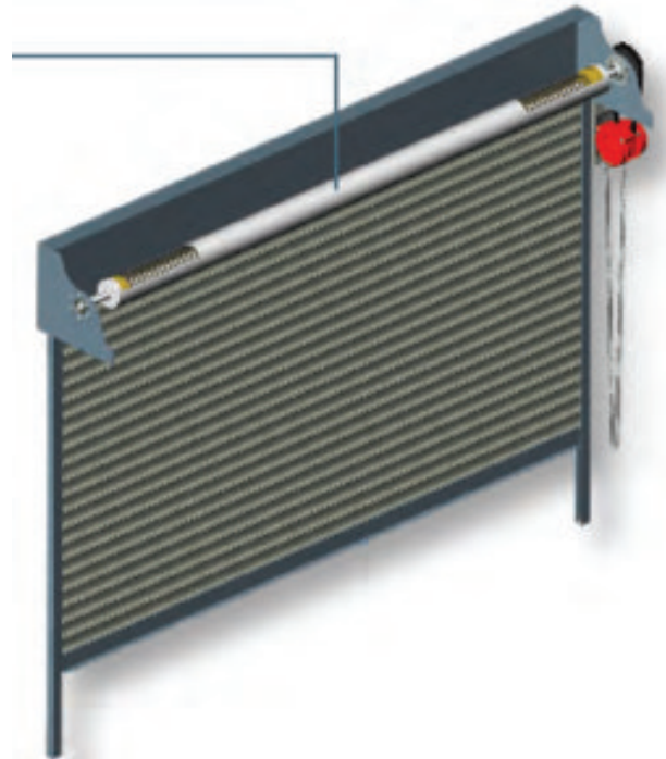
ตัวอย่างการติดตั้งประตูเหล็กม้วนระบบรอกโซ่ Rolling Shutter Installation of Chain Operation
