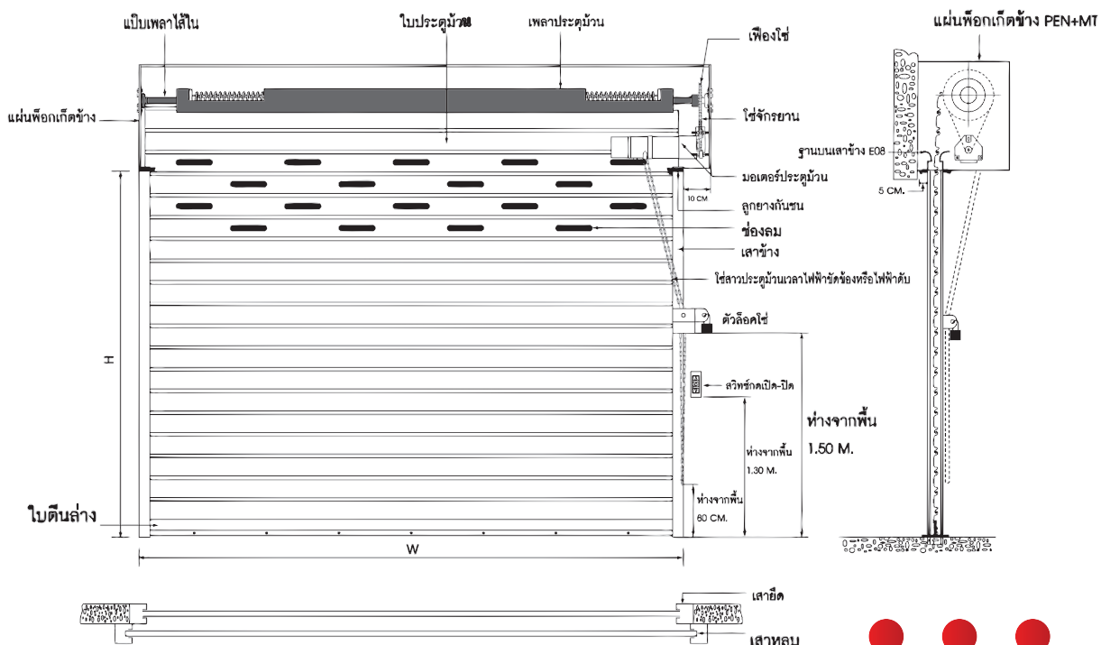
ตัวอย่างการติดตั้งประตูเหล็กม้วนระบบมอเตอร์ Rolling Shutter Installation of Motor Operation
