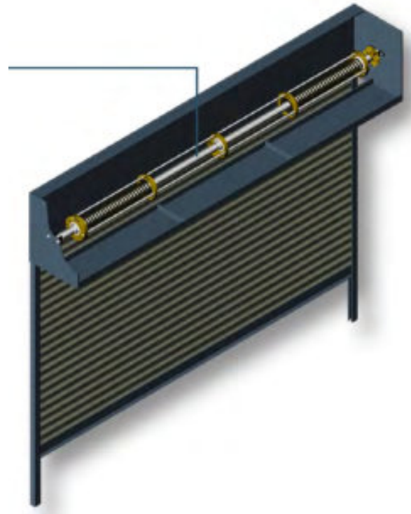
ตัวอย่างการติดตั้งประตูม้วนแบบมือดึง Manual Operation of Rolling Shutter Installation
