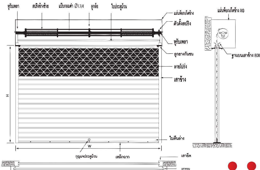
ตัวอย่างการติดตั้งประตูม้วนแบบมือดึง Manual Operation of Rolling Shutter Installation
